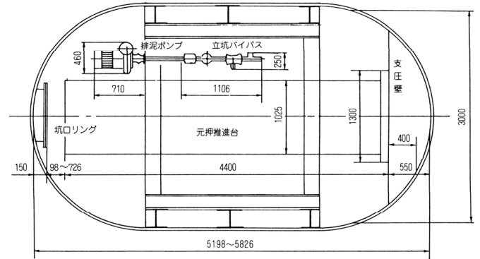
図 3-8 呼び径 350~500
