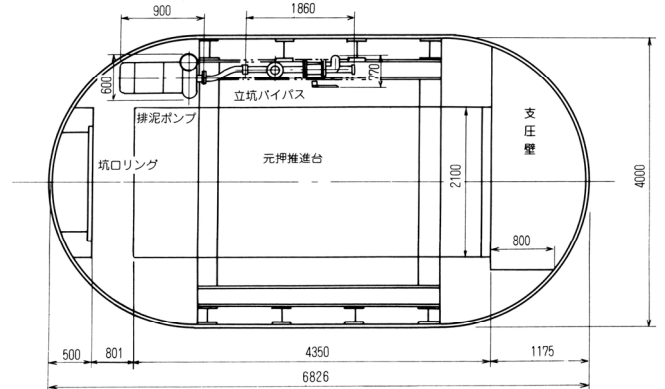
図 3-10 呼び径 900、1000
