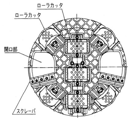
A 矢視
