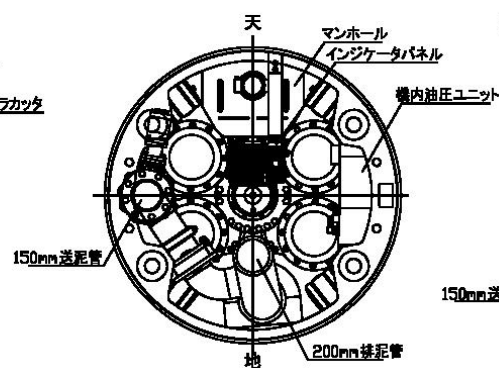
B ~ 断面
