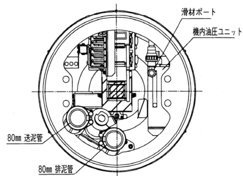
B 矢視
