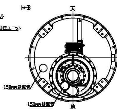
C ~ 断面
