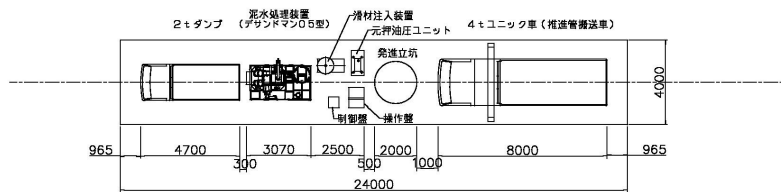
アングルモールドV工法 プラントヤード参考図 管呼び径φ200~φ400mm
