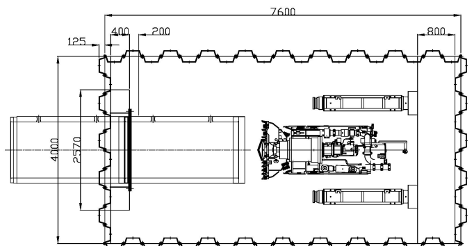
HP1200 普通土 多段ジャッキ (引戻し時時) 立坑内残管最大
