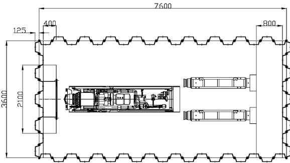
HP800 多段ジャッキ (発進時)
